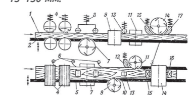
Четырёхсторонний строгальный станок C16-42 (Боровичский ЗДС) Предназначен для профильного строгания заготовок толщиной до 100 мм и шириной до 160 мм. Максимальная скорость подачи 26 м/мин.
