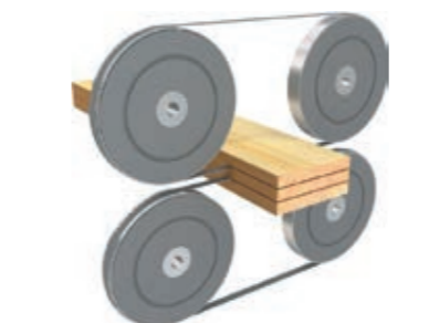
Ленточно-делительный станок HP-68 (High Point) Предназначен для раскроя досок. Доску 44–50 мм может раскроить по толщине на три доски для получения доски обшивки (вагонки) толщиной 12–14 мм.
