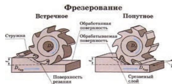
Рис. 1. Схемы встречного и попутного фрезерования заготовок
