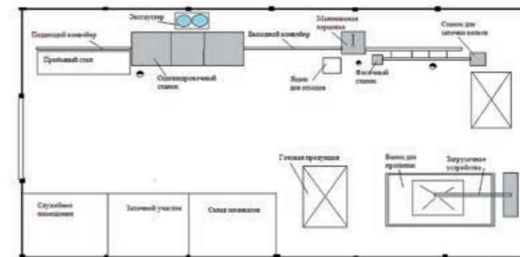
Рис. 7. Планировка цеха по переработке тонких лесоматериалов (18 x 9 м)
