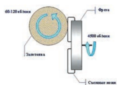
Рис. 2. Оцилиндровочный станок для тонкомера КБМ-200 (общий вид и схема обработки)
