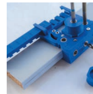
Рис. 5. Опрокидываемые кондукторы из пластика
