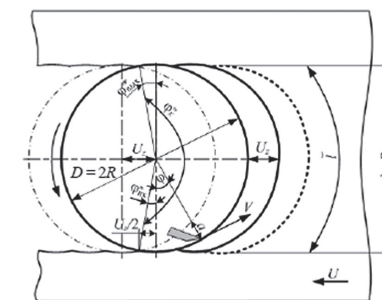
Рис. 3. Определение толщины стружки при закрытом фрезеровании (нестинге)
