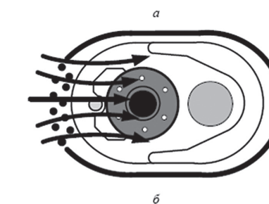
Рис. 4. Движение потоков воздуха в пылеприемниках: а – со щеточным основанием из щетины; б – с мягким основанием и при правильной аэродинамической конструкции приемника
